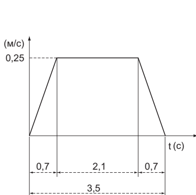
Диаграмма скоростей
