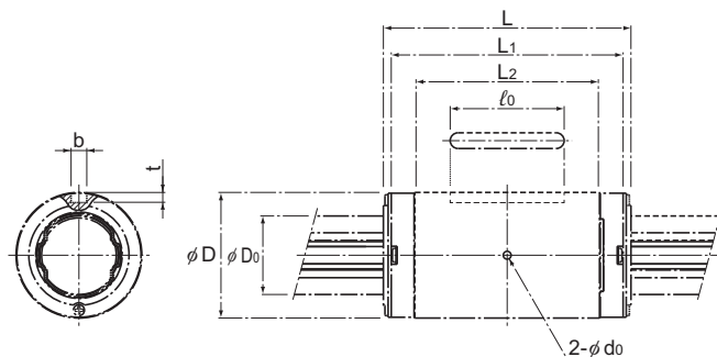
Модели LT10X...30X
