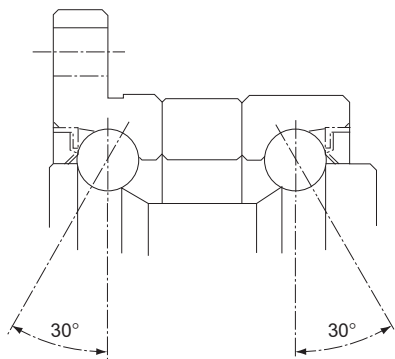
Модель LTR
