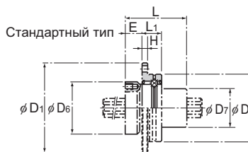
Модель LTR10A
