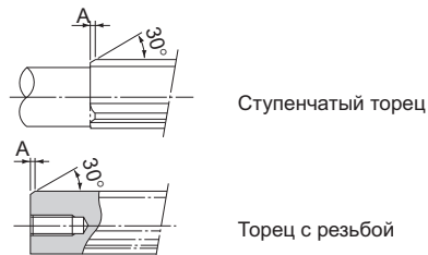
Рис.2 Фаска А
