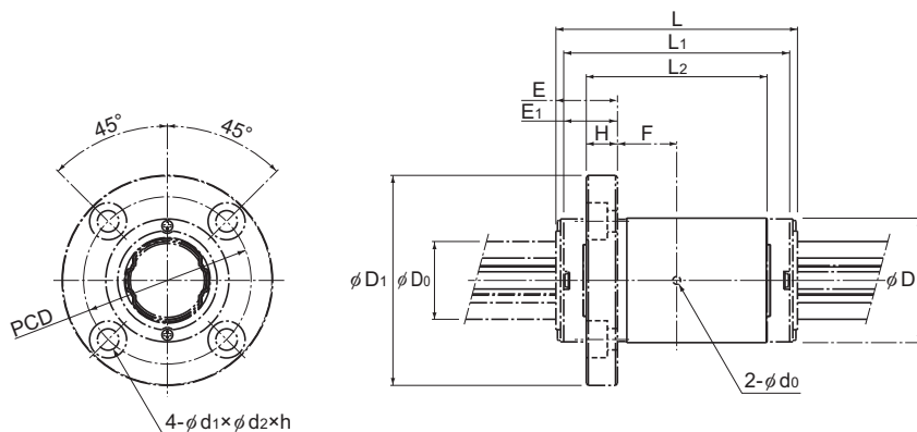
Модели LF10X...30X
